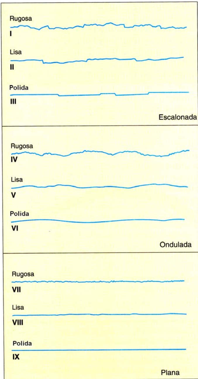
PERFIS DE RUGOSIDADE (ISRM, 1981)
